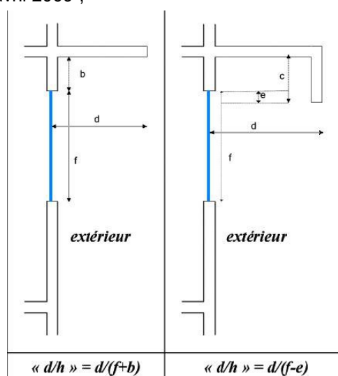
Figure 1 : « d/h » en cas de baie non libre
