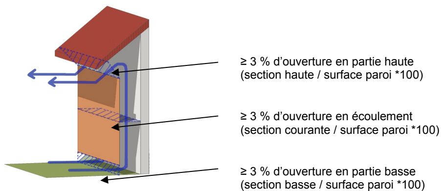
Figure 3 : pare-soleil ventilé (cf. annexe III – 3.3 2° de l'arrêté du 17 avril 2009)
