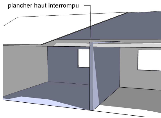
Figure 3 : le plancher haut présente un indice d'affaiblissement R_w + C supérieur à 35 dB
