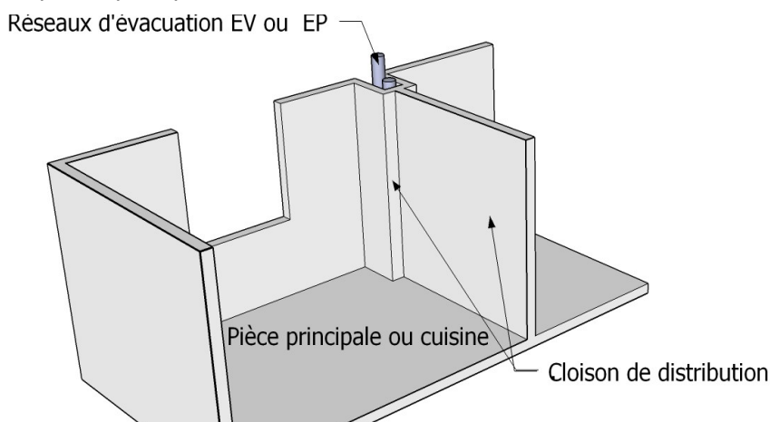
Figure 10 : exemple de disposition des réseaux d'évacuation extérieure à une pièce principale ou une cuisine
