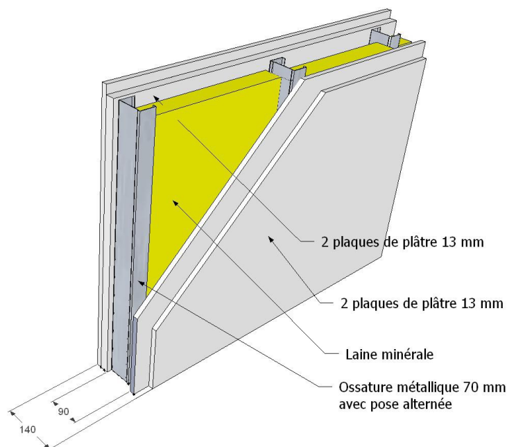
Figure 1 : exemple de paroi légère (répondant au principe de fonctionnement des parois multiples) satisfaisant aux exigences acoustiques concernant les parois séparatives verticales entre logements différents et également entre pièces principales, cuisines ou salle d'eau d'une part et locaux d'activité ou dépendances d'autre part
