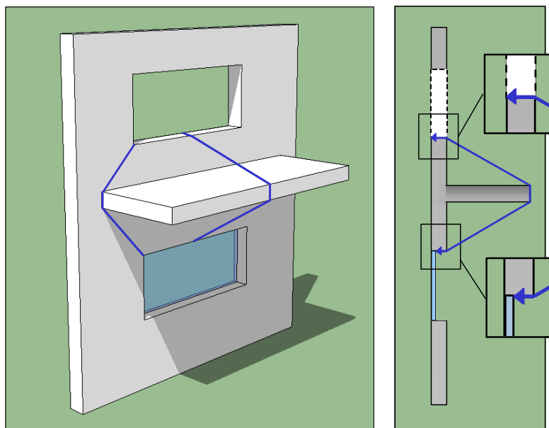
Figure 6 : distance déployée entre deux baies
