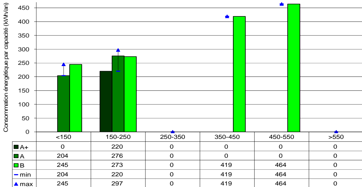
Figure 82 : Consommations énergétiques moyennes et extrêmes des congélateurs
